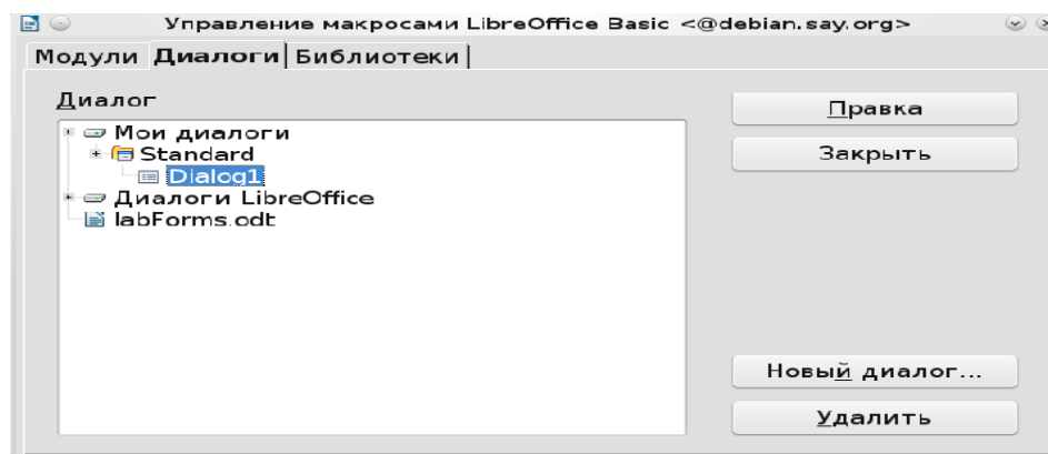
Рисунок 48 - Создание Диалога
