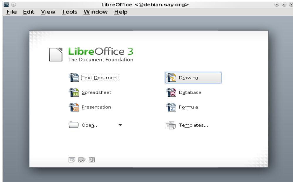
Рисунок 1 - LibreOffice
