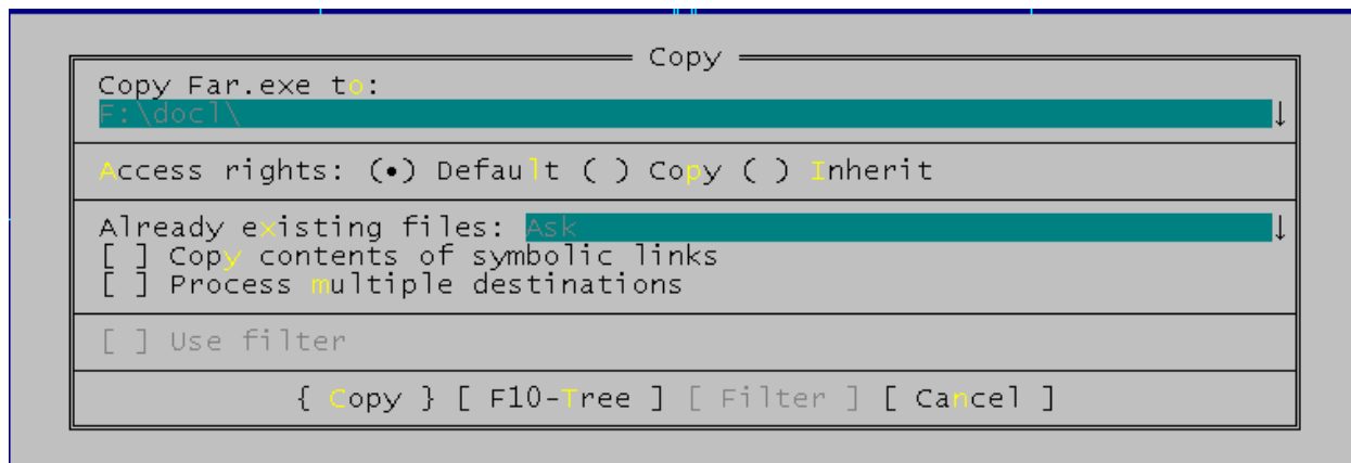
Рисунок 40 - Копирование файла
