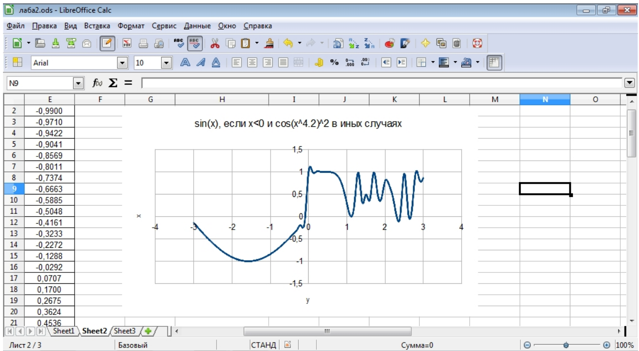
Рисунок 20 – Первый график.
