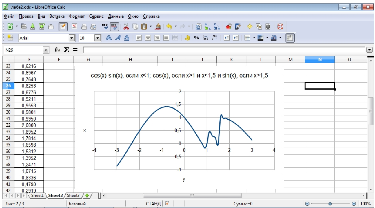
Рисунок 21 – Второй график.
