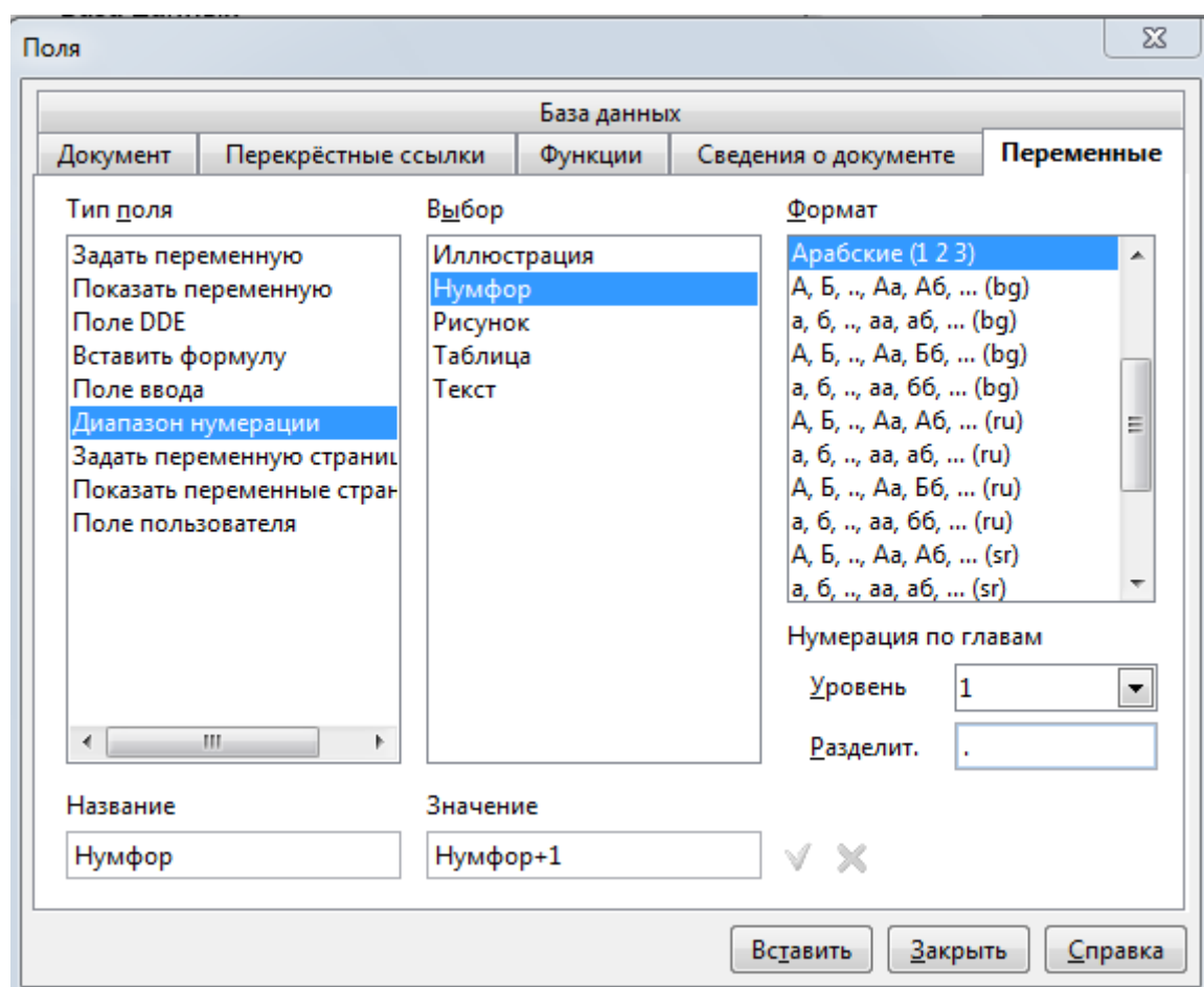
Рисунок 44. Окно редактирования
