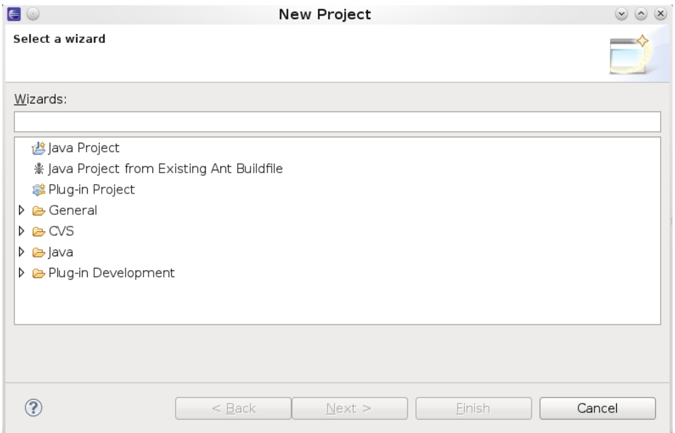
Рисунок 61 - Выбор проекта
