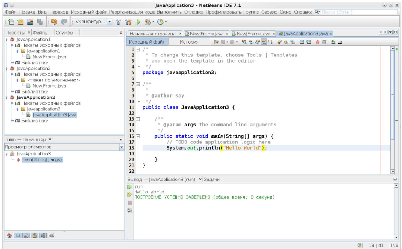
Рисунок 68 - Консольное приложение
