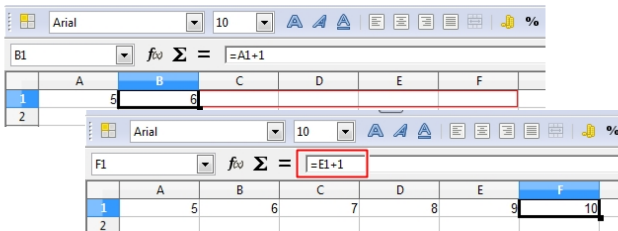
Рисунок 5 – Копирование формулы
