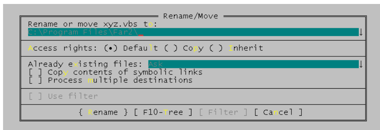
Рисунок 41 - Переименование файла
