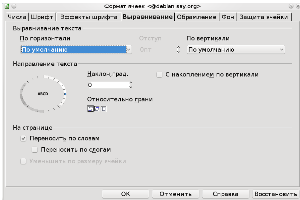
Рисунок 25 - Форматирование ячейки
