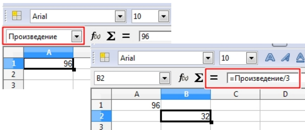
Рисунок 4 – Имя ячейки
