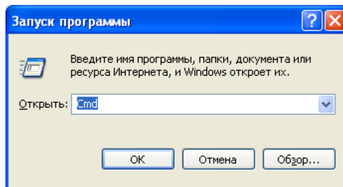
Рисунок 34 - Запуск программ
