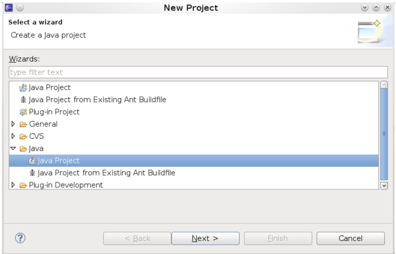
Рисунок 62 - Создание проекта
