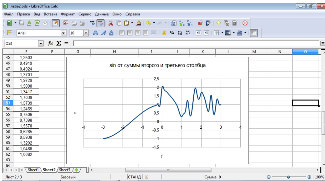
Рисунок 22 – Третий график.
