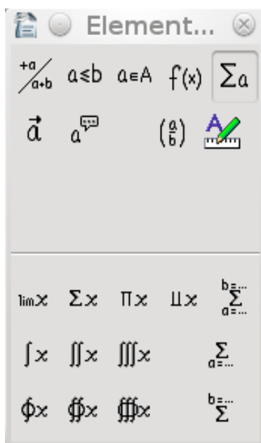
Рисунок 15 - Редактирование формулы
