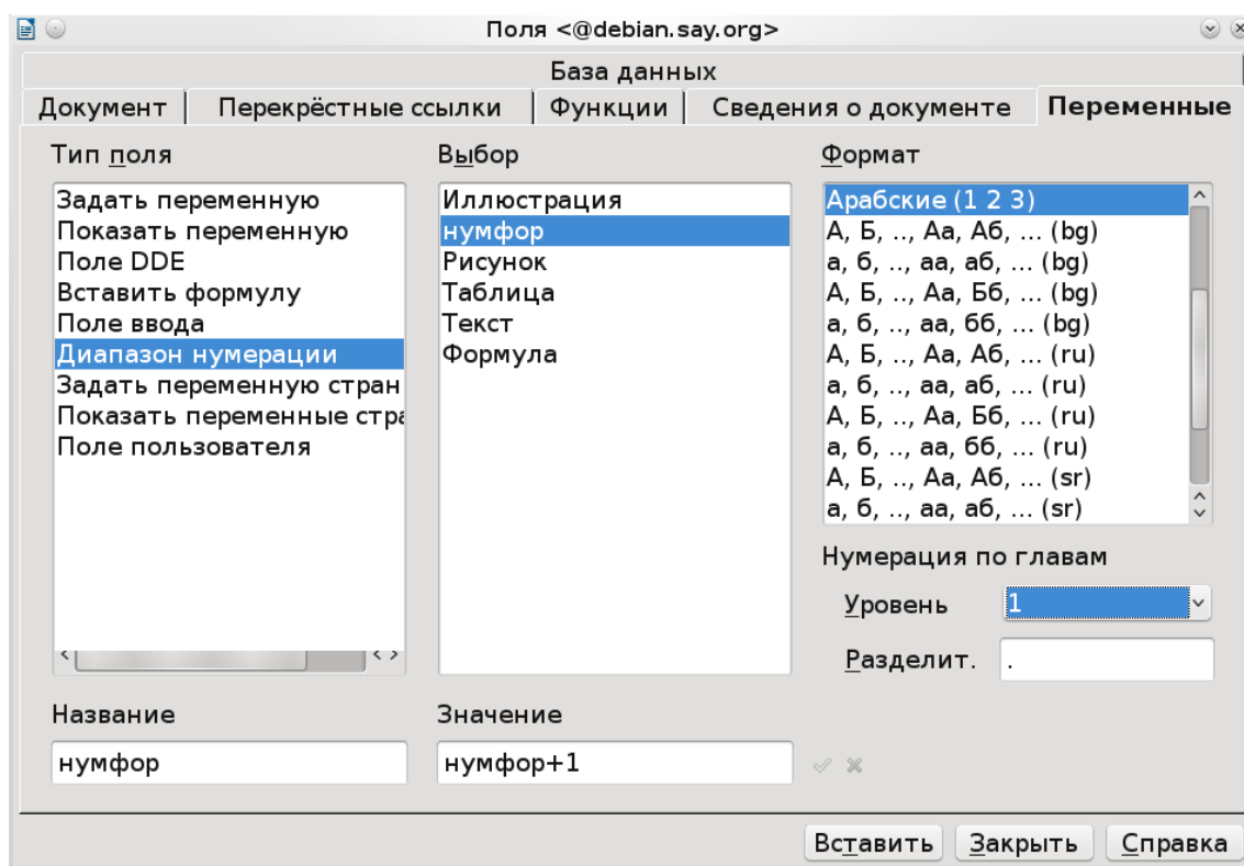
Рисунок 16 - Настройка поля
